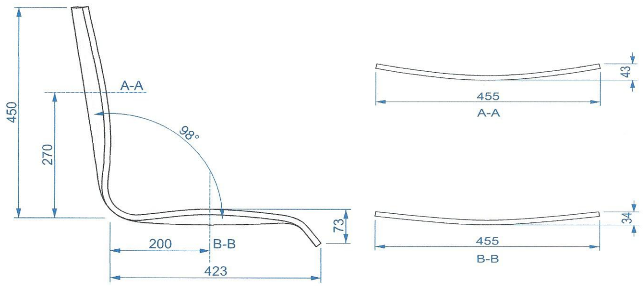
Plano básico cotas orientativas en mm.
